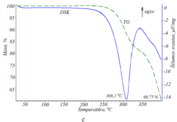
4 pav. Vienlaikės terminės analizės (DSK/TG) kreivės: a – AS (N.T.), b – AS (Gr.), c – AS (Nov.), d – MOP (BK.f.)
