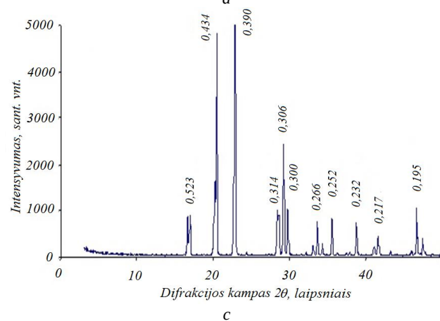
5 pav. Rentgeno difrakcinės analizės kreivės: a – AS (N.T.), b – AS (Gr.), c – AS (Nov.), d – MOP (BK.f.)
