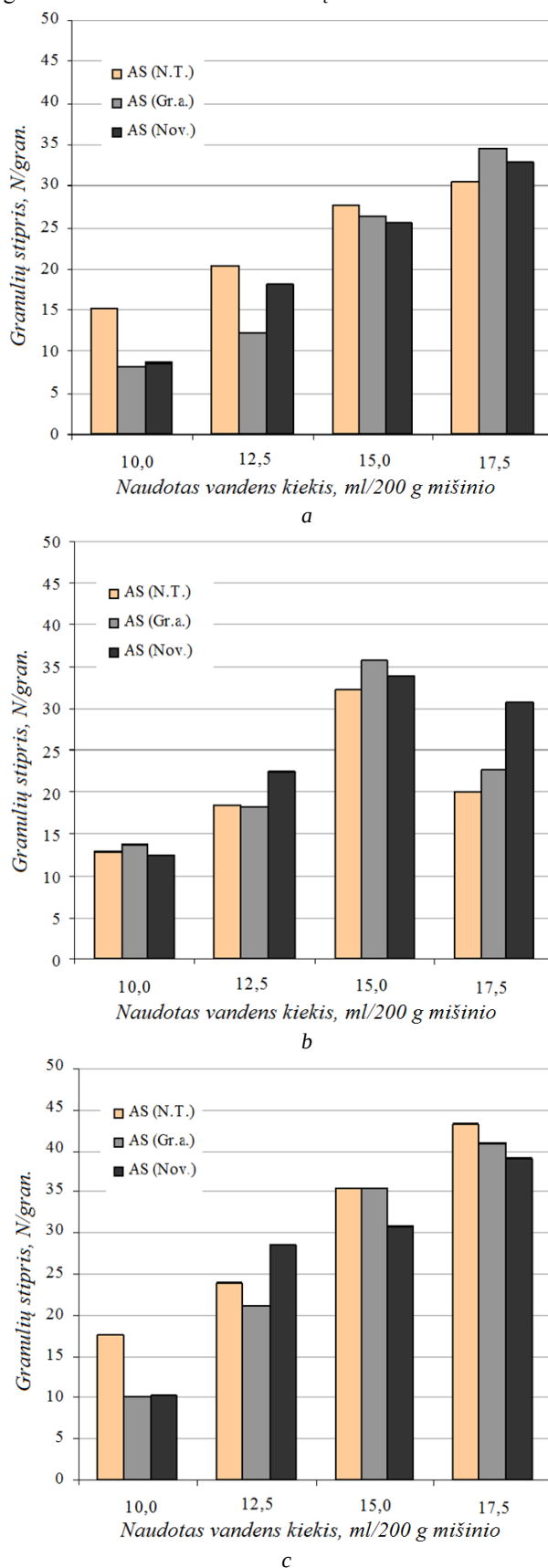
9 pav. Statinio granulių stiprio priklausomybė nuo žaliavų mišinio drėgmės, esant skirtingos kilmės AS ir MOP (BK.f.), kai returo kiekis: a – 0 %; b – 10 % ir c – 20 %
