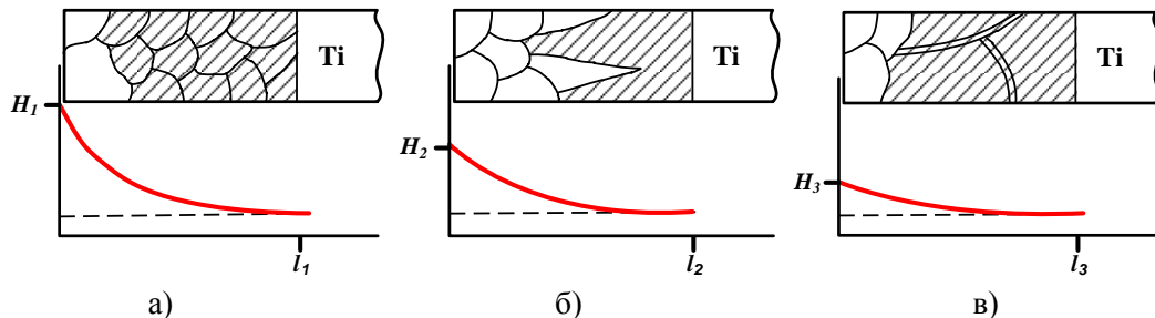
Рисунок 3. – Загальні закономірності формування газонасичених шарів на титанових сплавах різних структурних класів: а – \alpha - і псевдо- \alpha , б – \alpha+\beta , в б – \beta
