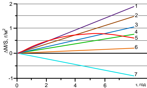
Рисунок 2. – Кінетика зміни маси зразків титанових сплавів BT1-0 (1), ОТ4-1 (2, 7), BT5-1 (3, 5), ПТЗВ (4) і BT6с (6) під час витримки за температури 900°C (1, 2, 3, 4, 6, 7) і 1000°C (5) в газовому середовищі тиском 1,33 мПа (1, 3, 4, 5, 6, 7) і 13,3 мПа (2).
