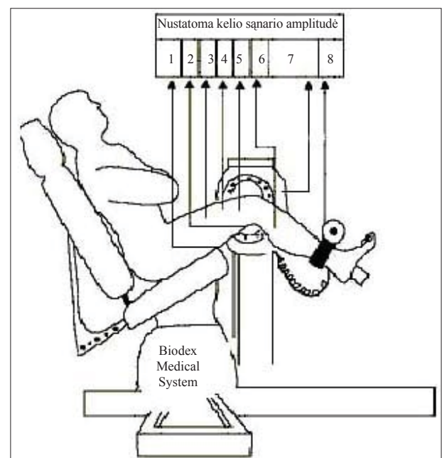
1 pav. Izokinetinio dinamometro veikimo schema
