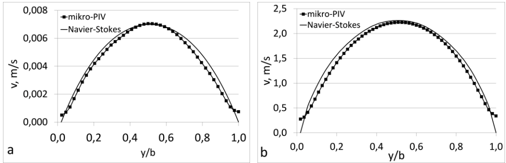
2.7 pav. Eksperimentinių ir teorinių greičio profilių tiesiame kanale palyginimas, kai a) Re_{Dh} = 1,7 ir b) Re_{Dh} = 600
