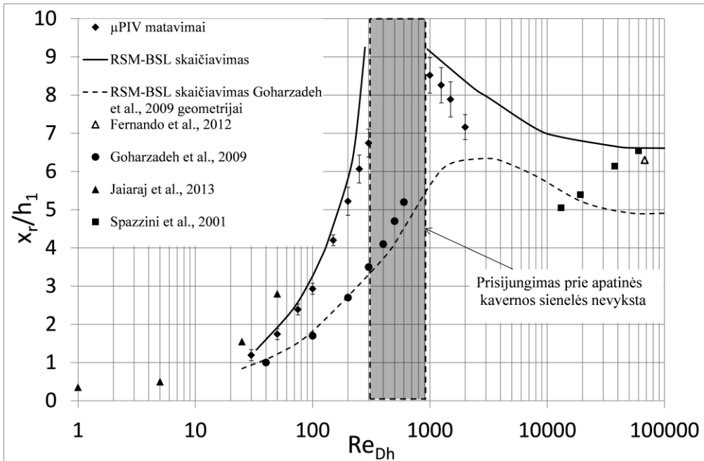
3.7 pav. Eksperimentinių ir sumodeliuotų recirkuliacinės zonos ilgio verčių palyginimas tarpusavyje ir su kitų autorių rezultatais
