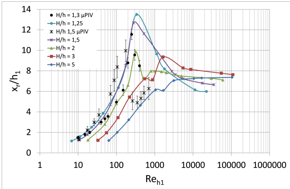
3.19 pav. Recirkuliacinės zonos ilgio priklausomybė nuo Re_{h1} pereinamojo tipo kavernoje ( L/h_1 = 16 ) esant skirtingiems kanalo išplatėjimo santykiams
