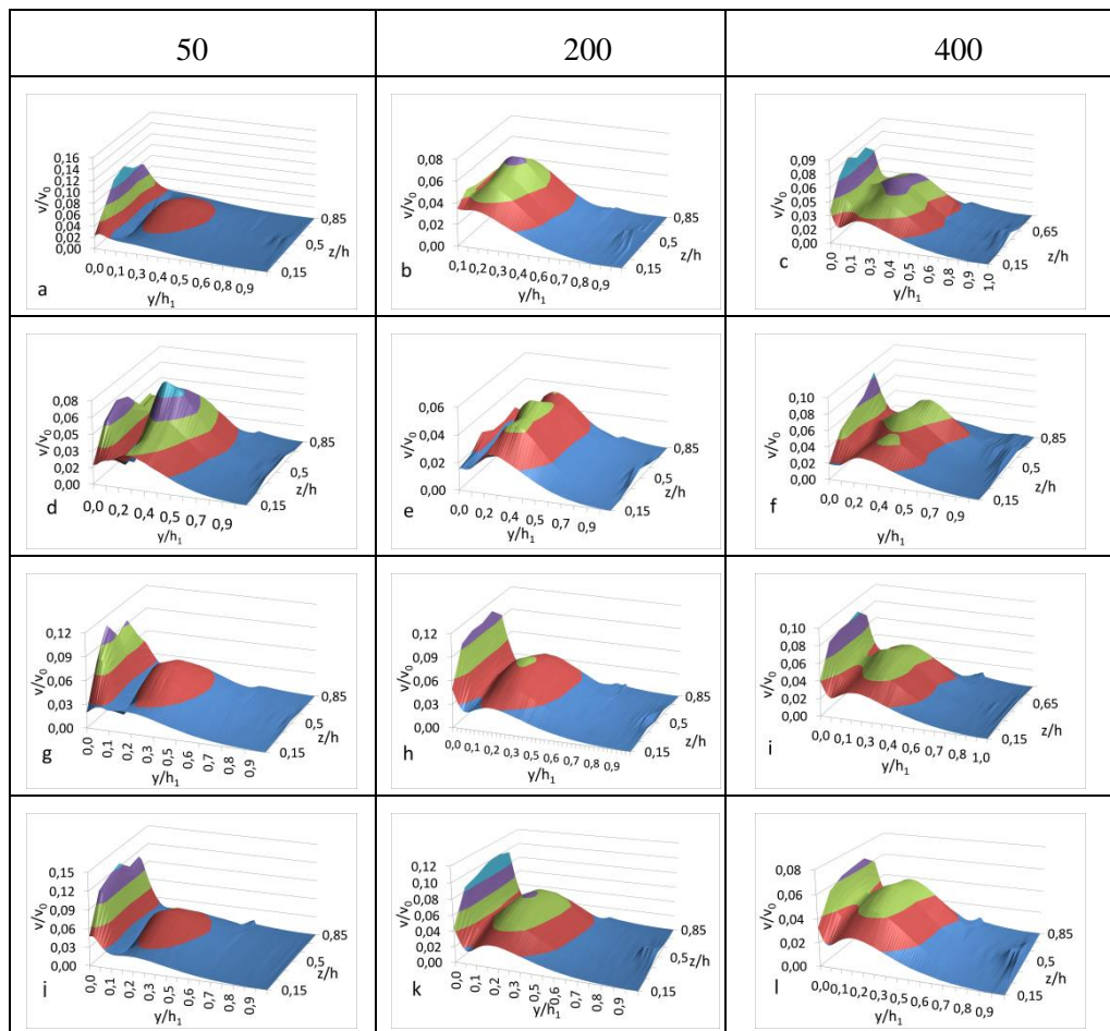
3.39 pav. Erdvinis greičio pasiskirstymas kanalo ašyje esant skirtingoms tekėjimo kanale sąlygoms: a) b) c) – stacionarus tekėjimas, d) e) f) – Wo_{Dh} = 0,6 , g) h) i) – Wo_{Dh} = 2,0 ir i) j) k) – Wo_{Dh} = 6,3
