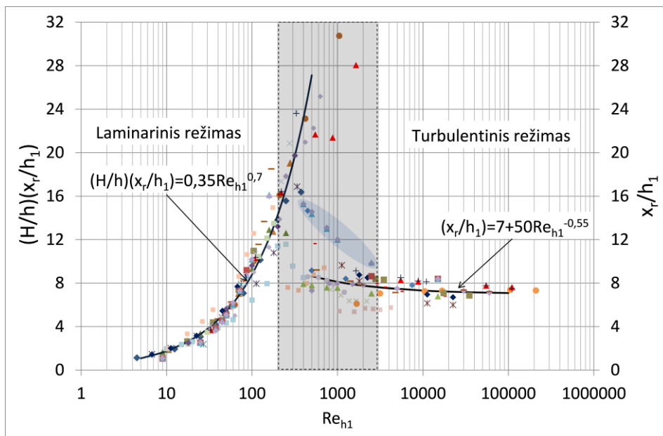
3.21 pav. Recirkuliacinės zonos ilgio priklausomybės nuo Re_{h1} apibendrinimas laminariniame ir turbulentiame tekėjimo režimuose
