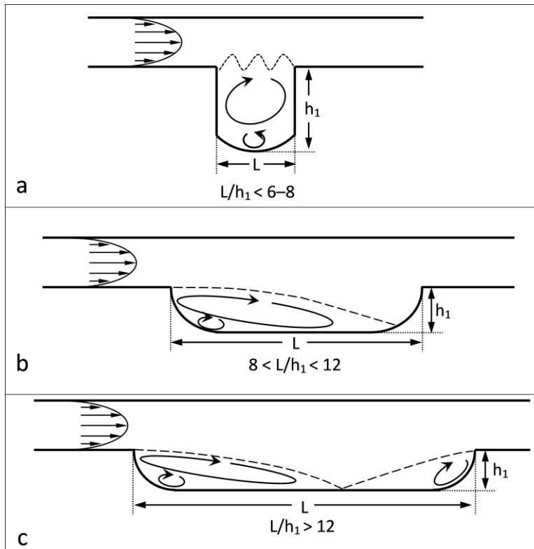
1.4 pav. Kavernų klasifikacija pagal kavernos ilgio ir gylio santykį ( L/h_1 ) ir tekėjimo struktūra kavernose. a) atvirojo tipo, b) pereinamojo tipo ir c) uždarojo tipo kaverna
