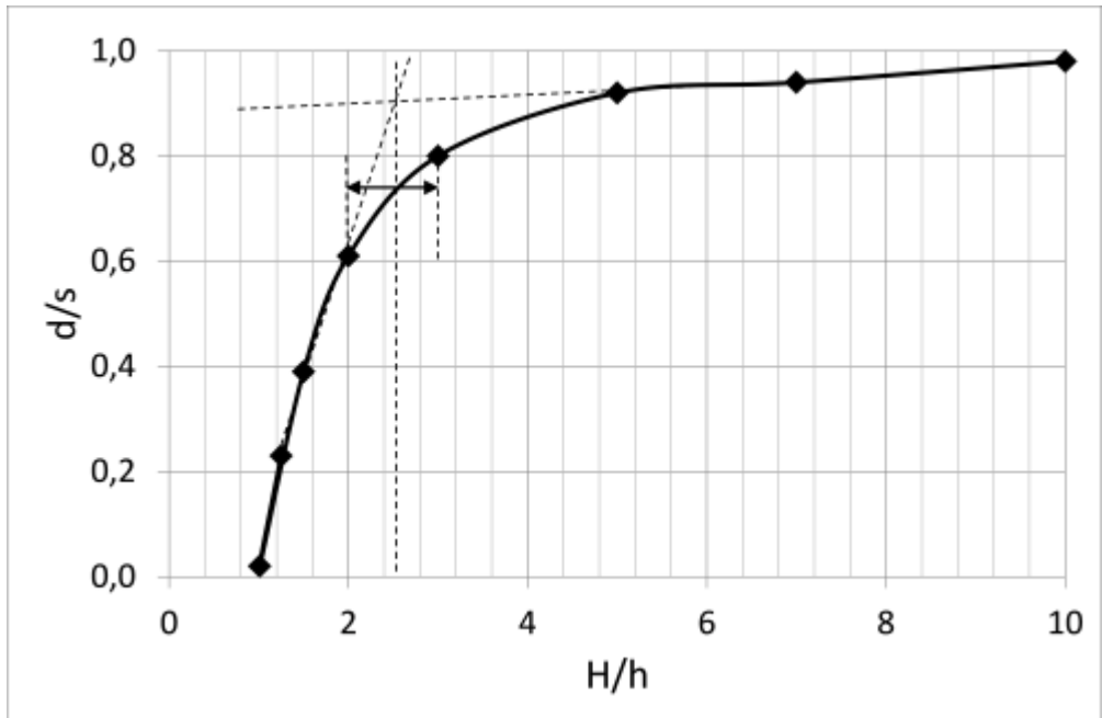
3.14 pav. Maišymosi sluoksnio kavernoje plėtimosi priklausomybė nuo kanalo išplatėjimo santykio
