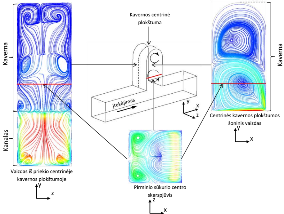
3.36 pav. Srauto linijos skirtingose kavernoje plokštumose
