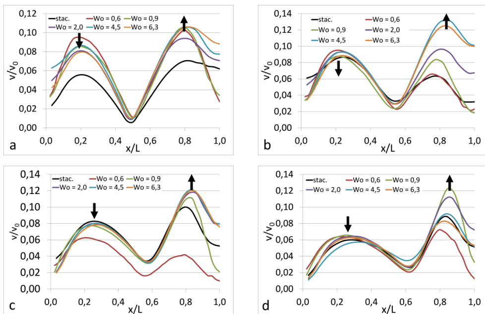
3.38 pav. Santykinio greičio profiliai per pirminio sūkurio centrą centrinėje matavimo plokštumoje esant skirtingoms tekėjimo sąlygoms a) – Re = 50 , b) Re = 100 , c) Re = 200 , d) Re = 400
