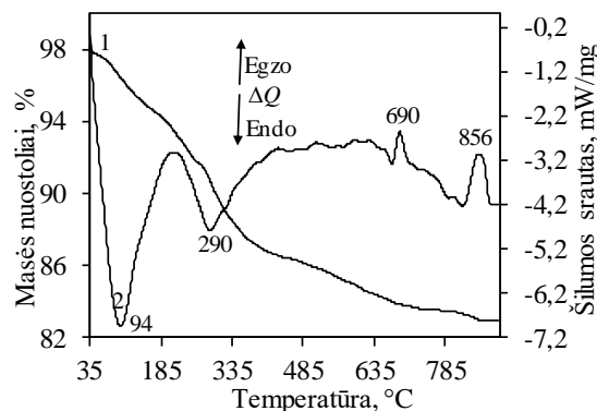
6 pav. Hidroterminės sintezės ( C/S=1,5 ; A/S+A=0,05 , 200\text{ }^\circ\text{C} ) produktų TGA (1 kr.) ir DSK (2 kr.) kreivės \text{CaO}\text{-SiO}_2\text{-Al}_2\text{O}_3\text{-H}_2\text{O} sistemoje, kai priedas \text{Cr}(\text{NO}_3)_3 , o izoterminio išlaikymo trukmė 24 h
