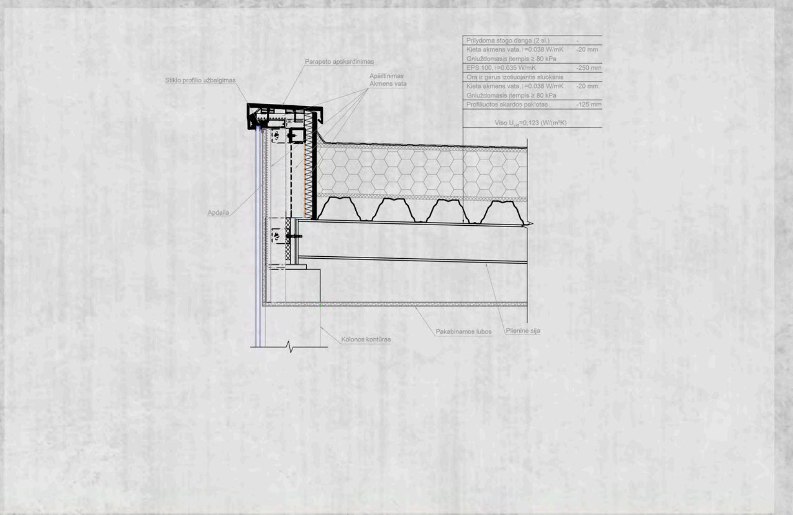
DETALĖ 3 M:20
