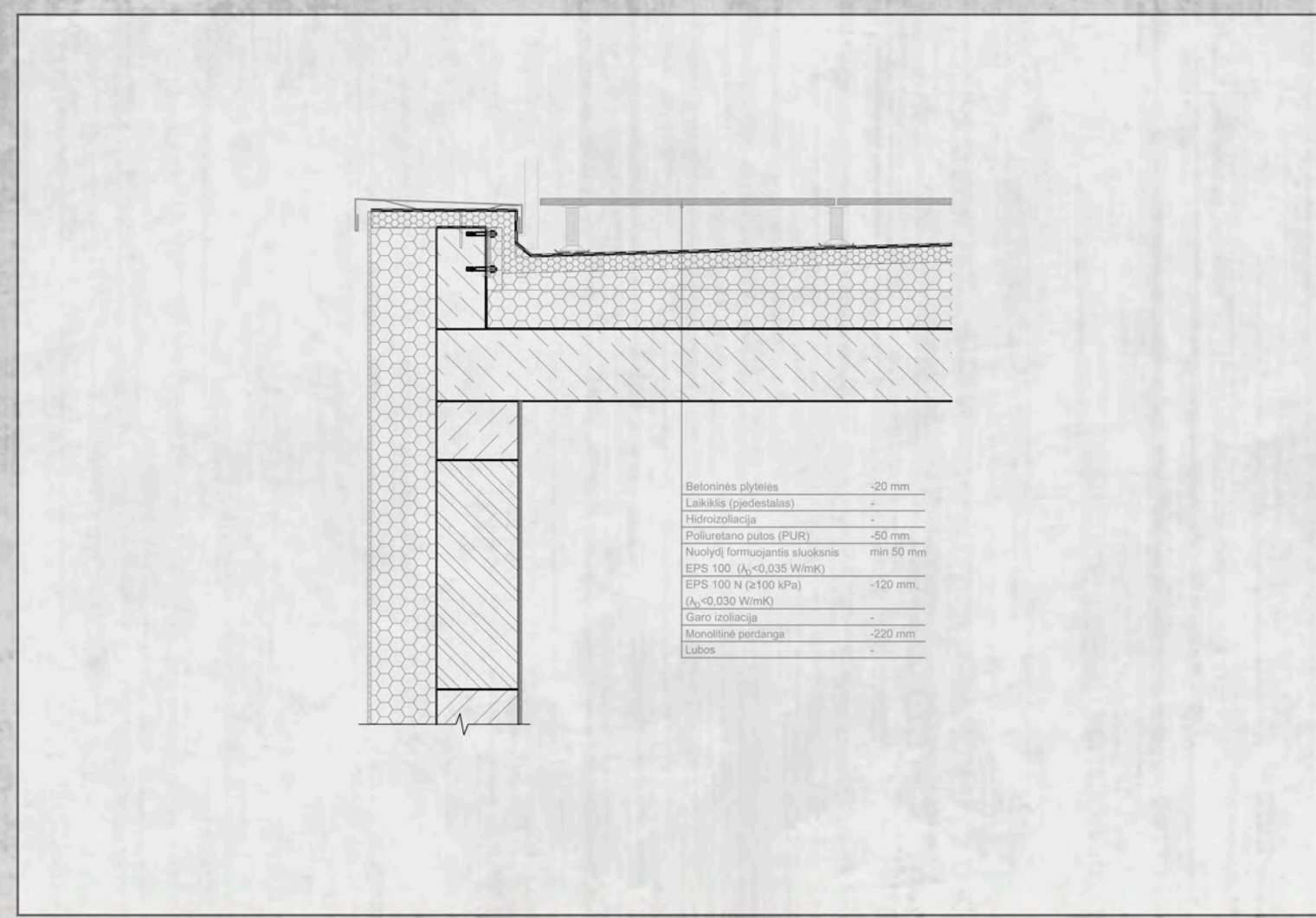
DETALĖ 2 M:20
