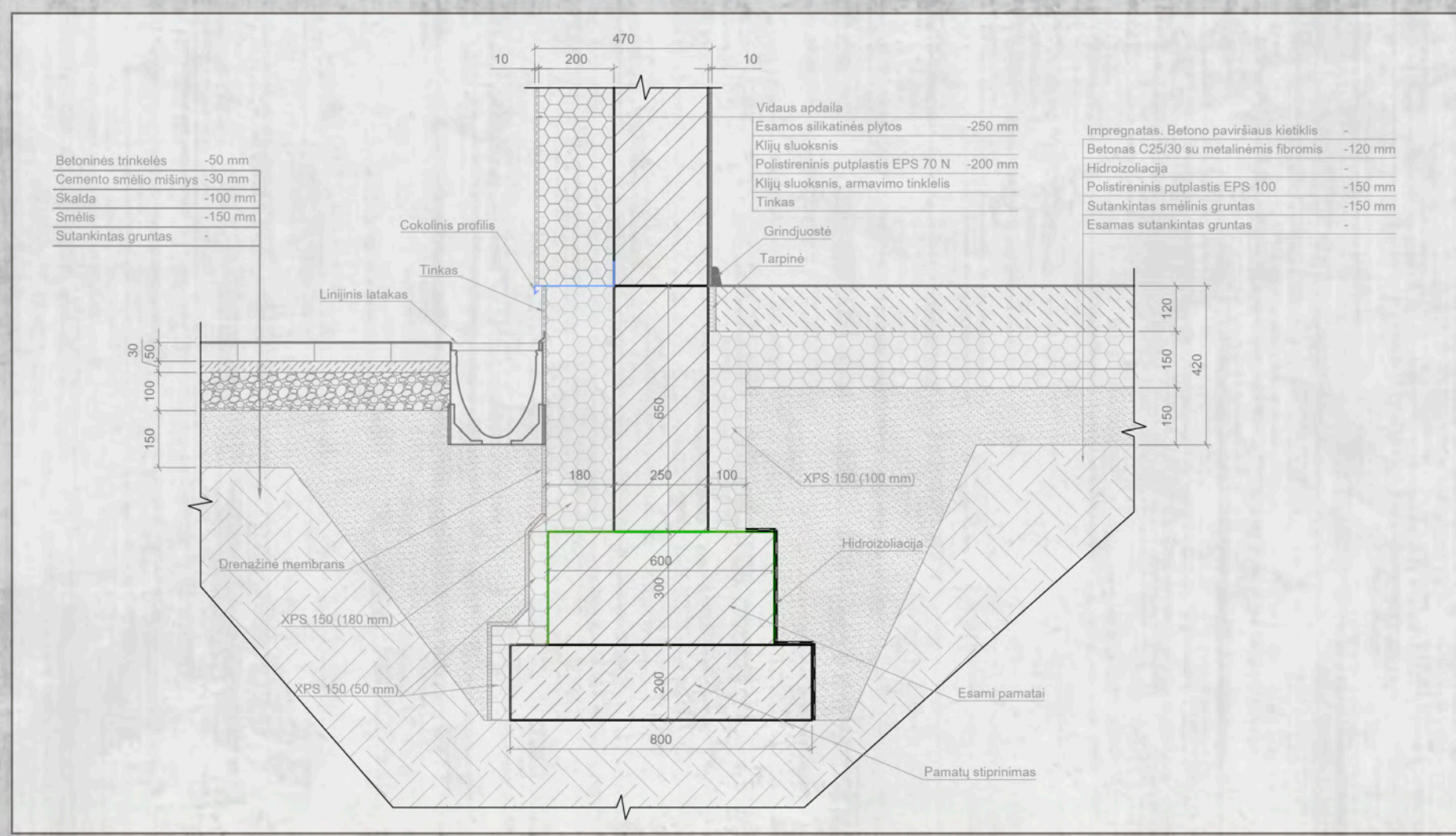
DETALĖ 1 M:20
