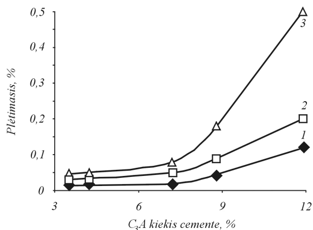
7 pav. Cementinių skiedinių ( C/S = 1:4 ; V/C = 0,6 ) plėtra, %, po 3 (1), 4 (2) ir 6 (3) mėn. laikymo 5 % Na_2SO_4 tirpale [1]
