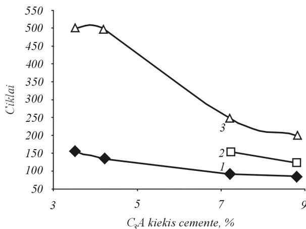
6 pav. Cementinių skiedinių ( C/S = 1:4 ; V/C = 0,6 ) atsparumo šaldymui ir mirkymui 5 % Na_2SO_4 tirpale priklausomumas nuo C_3A kiekio cemente: 1 ir 2 – su 25 % opokos priedu, 3 – 5 % NaCl tirpale (1 ir 3 – C_3A = 8,8\% , 2 – C_3A = 7,1\% )
