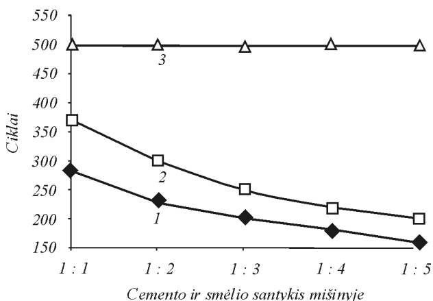
3 pav. Įvairios mineralinės sudėties cementų skiedinių atsparumas šalčiui ir 5\% NaCl tirpalo cikliškam veiksmui: 1 – su 8,8\% , 2 – su 7,1\% C_3A . Skiediniai su 4,2 ; 3,8\% C_3A bei su opokos priedu nesuiri iki 500 šaldymo ciklų (3 kr.)
