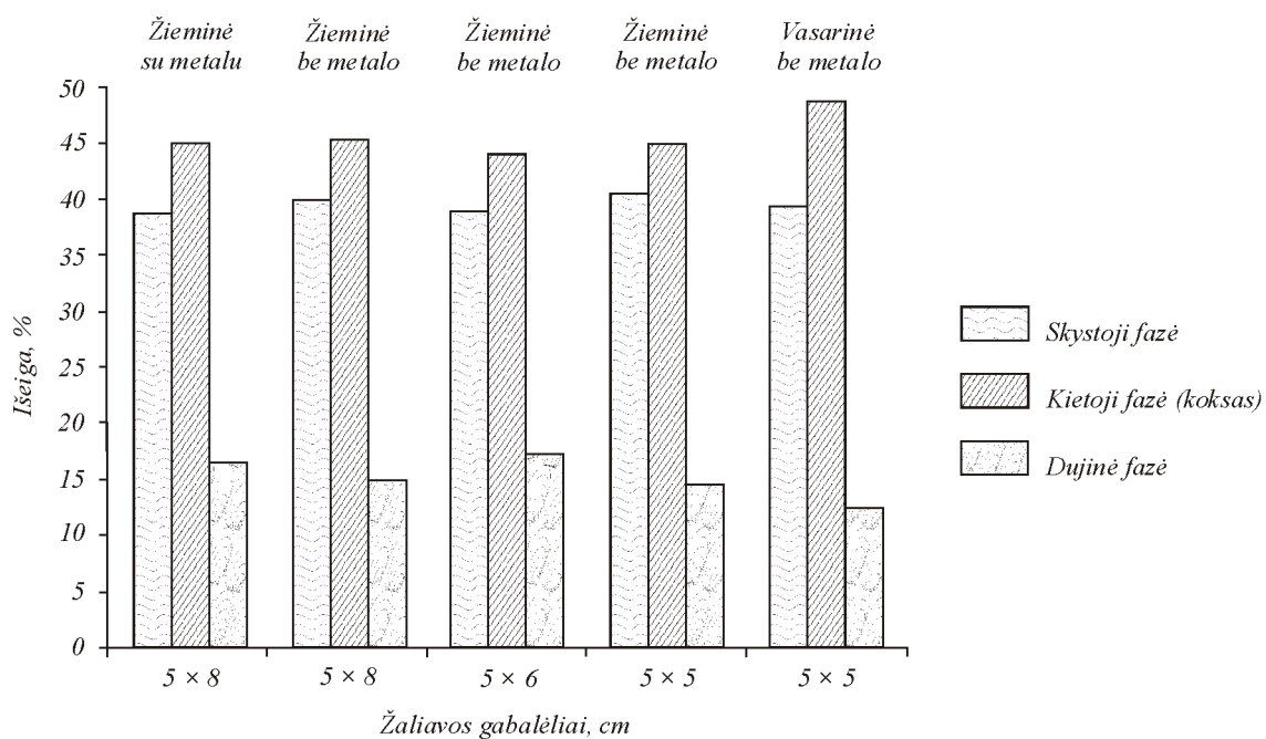
3 pav. Padangų pirolizės produktų išeiga
