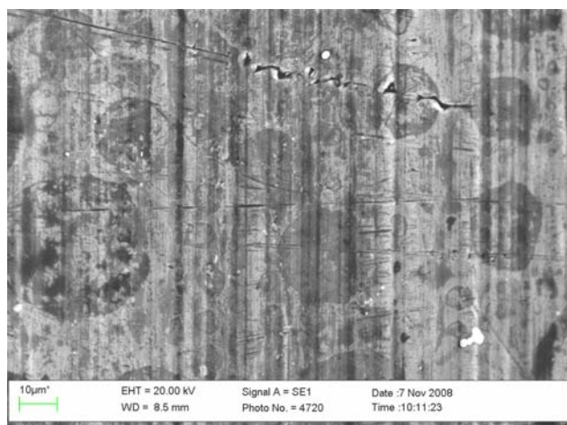
Al K 2
