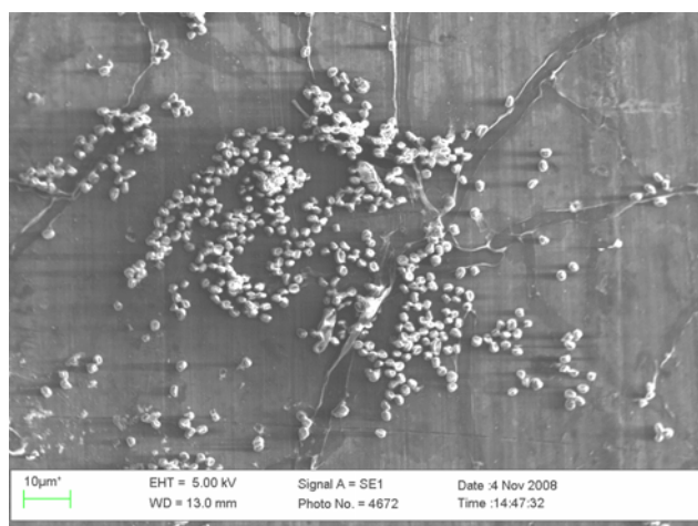
Al I 4
