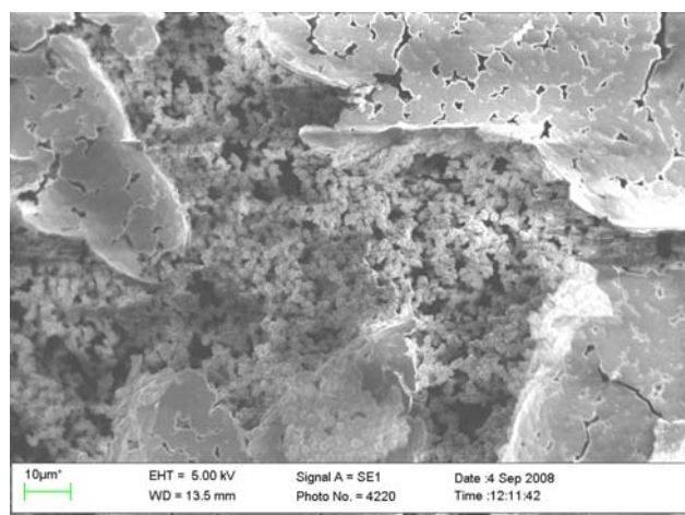
Fe 1
