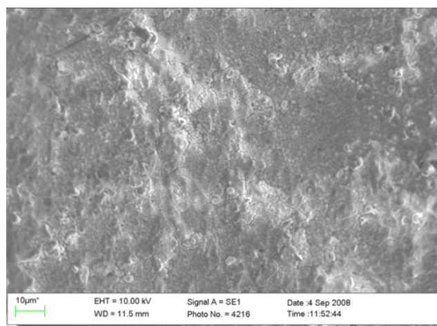
Fe K 2
