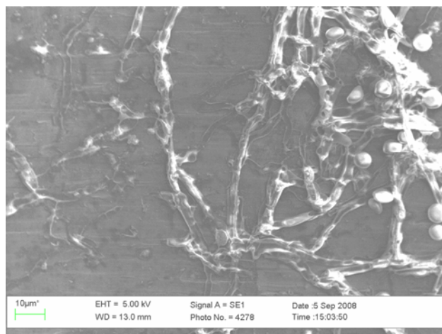
Al I 3
