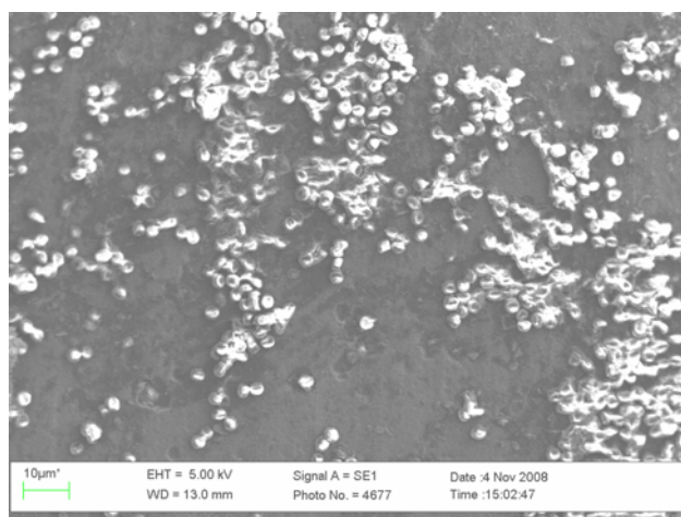
Al I 5
