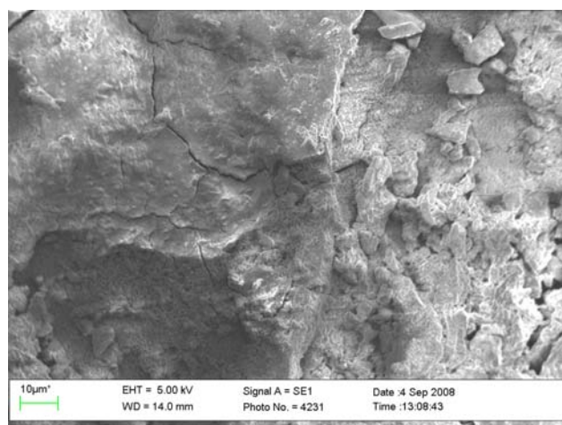
Fe 5
