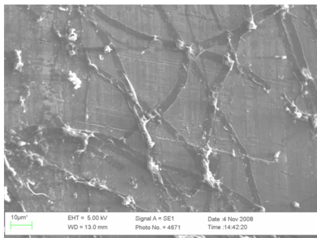
Al I 2
