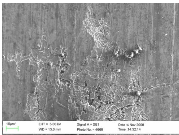
Al I 1
