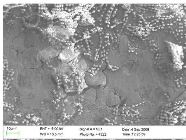
Fe 2
