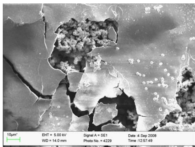
Fe 4
