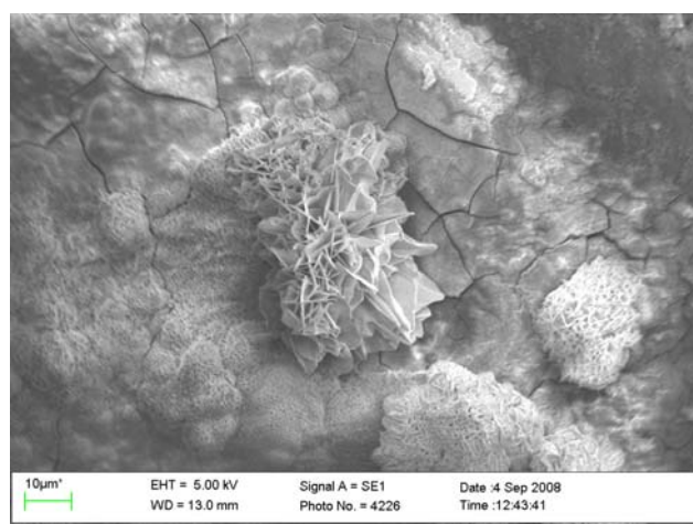
Fe 3
