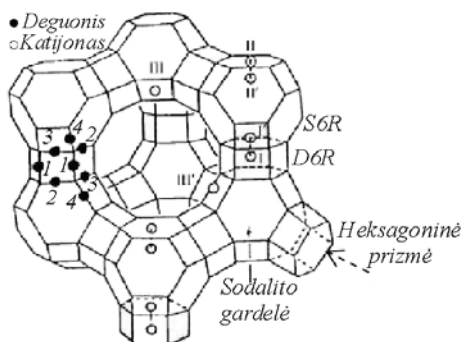
1 pav. Fožazito struktūra, kurioje aiškiai nurodytos keturios deguonis atomų buvimo vietos ir galimos katijonų pozicijos [19]
