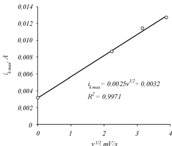
5 pav. i_{\text{max}} priklausomumas nuo v^{1/2} , kai Te(VI) koncentracija rūgščiajame manganavimo elektrolite 2,20 mmol/l
