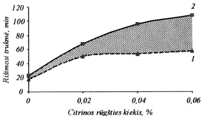
11 pav. Citrinės rūgšties įtaka gipso rišimosi trukmei: 1 – rišimosi pradžia; 2 – rišimosi pabaiga
