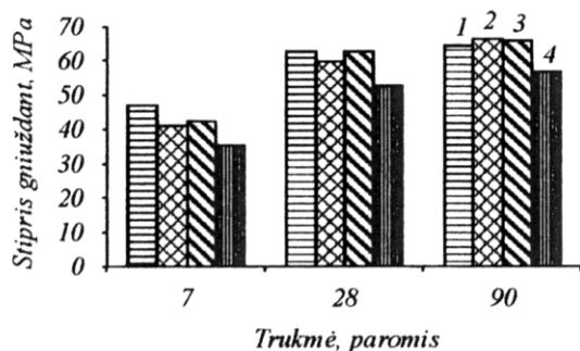
4 pav. Sukietėjusių portlandcemenčio bandinių stipris gniuždant. Bandinys: 1 – be priedo; 2 – su 5 % degtu kaolininio molio; 3 – su 10 % degtu kaolininio molio; 4 – su 20 % degtu kaolininio molio
