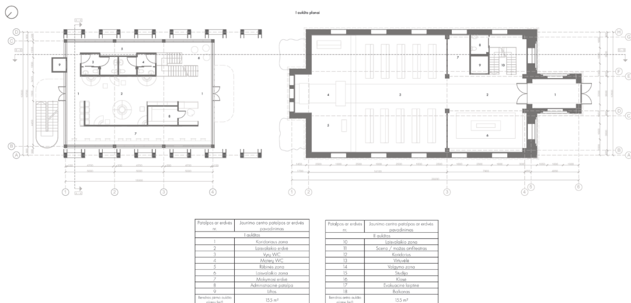
16 pav. Jaunimo centro ir Virbalio evangelikų liuteronų bažnyčios pirmo aukšto planai (sudaryta autorės)
