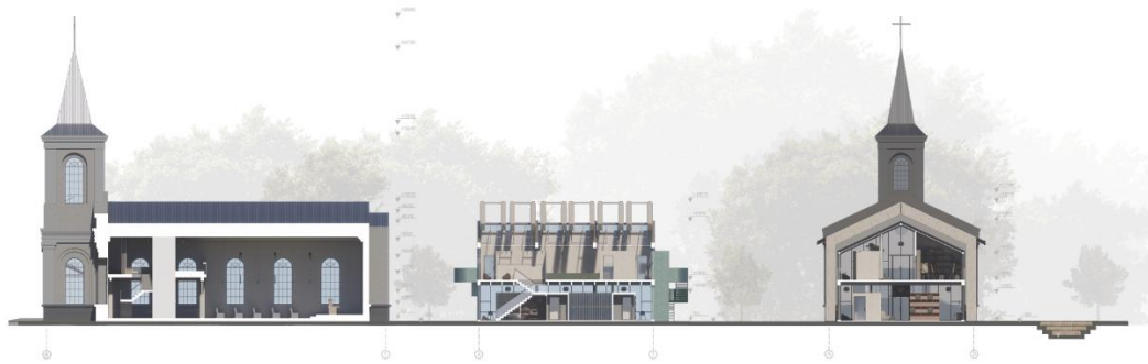
22 pav. Pjūviai (sudaryta autorės)
