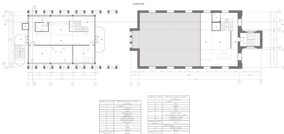
17 pav. Jaunimo centro ir Virbalio evangelikų liuteronų bažnyčios antro aukšto planai (sudaryta autorės)
