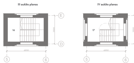
18 pav. Virbalio evangelikų liuteronų bažnyčios trečio ir ketvirto aukštų planai (sudaryta autorės)
