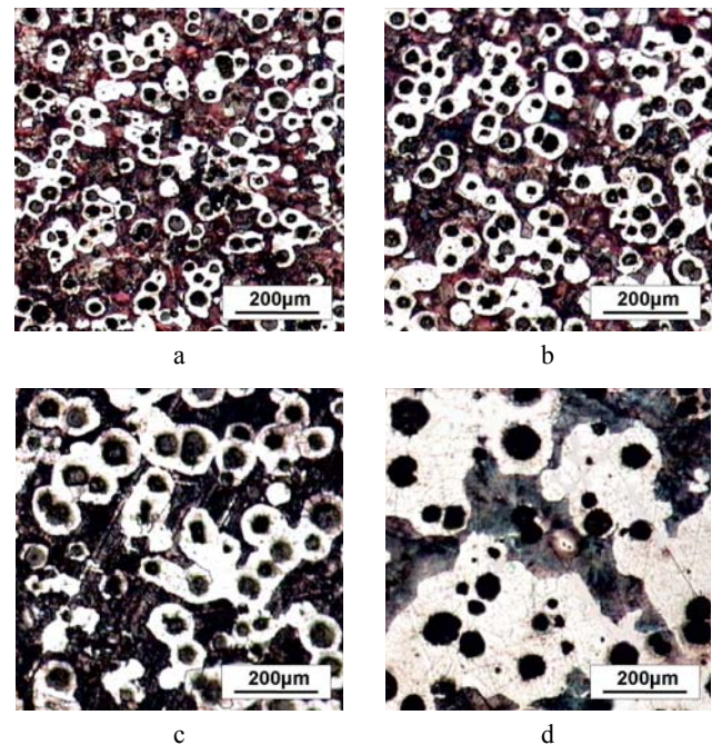
Fig. 5. Microstructure in the 3 (a), 5 (b), 10 (c) and 24 (d) mm plate castings
