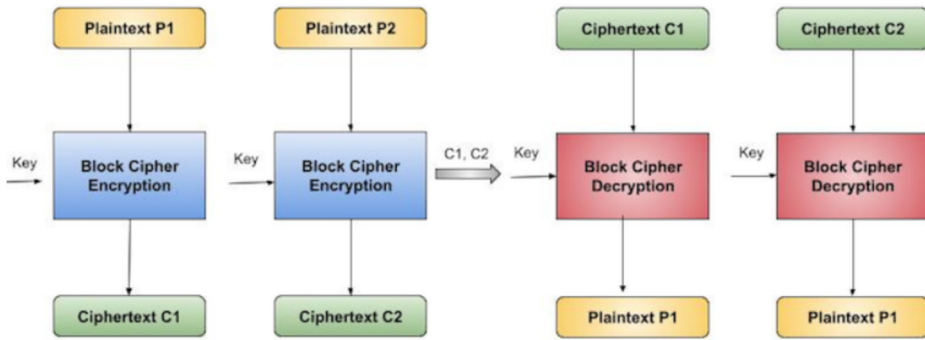
Fig. 1. ECB Mode.
