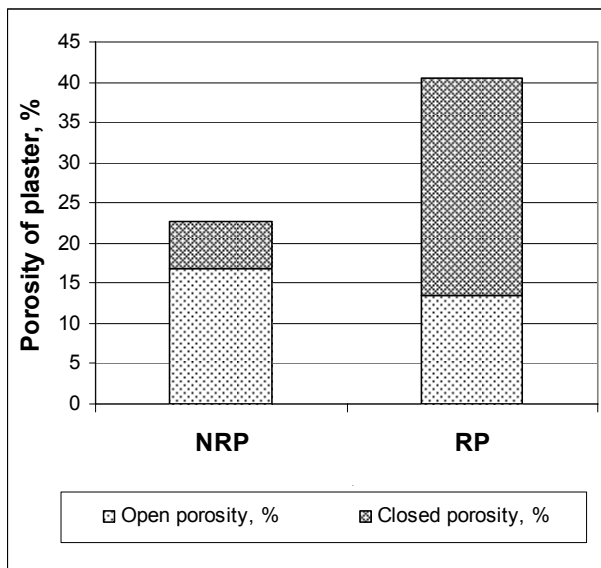
Fig. 8. Porosity parameters of plaster
