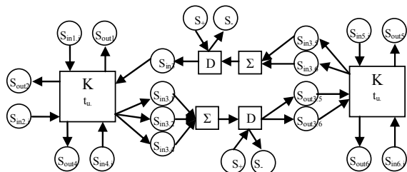
9 pav. Dviejų sankryžų srautų sujungimo schema
