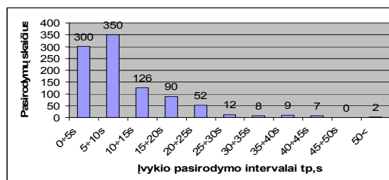
5 pav. Įeinančio įvykių srauto S_{in2} (K. Petrausko g. nuo Parodos kalno) pasirodymo visų intervalų histograma. Bendras įvykių skaičius 956
