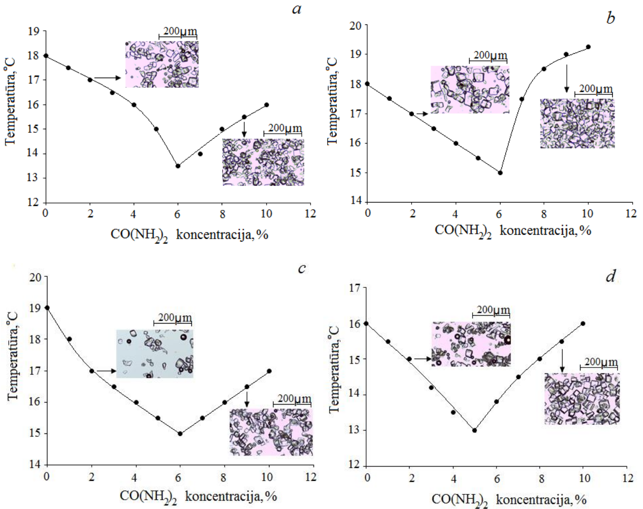
1 pav. PT, gautų esant \text{KCl} : \text{NH}_4\text{H}_2\text{PO}_4 = 0,8 : 0,2 ir konversijos temperatūrai: a – 20, b – 40, c – 60, d – 80 °C, kristalizacijos temperatūros priklausomybė nuo karbamido koncentracijos. KF optinės mikroskopijos nuotraukos.
