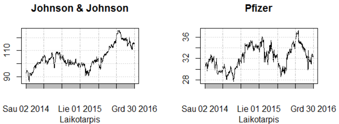
6.1. pav. Grynujų akcijų kainų laiko eilučių grafinis vaizdas
