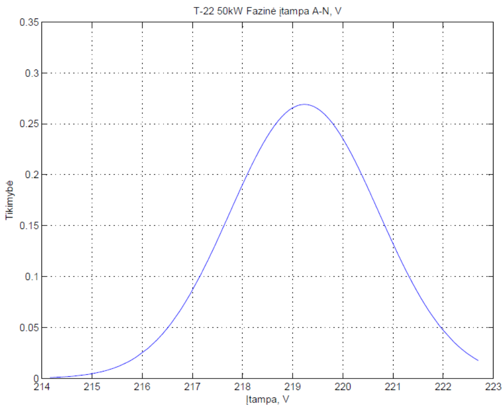
4.2.3 Pav. T-22 50 kW savų reikmių transformatoriaus normalusis (Gauso) skirstinys
