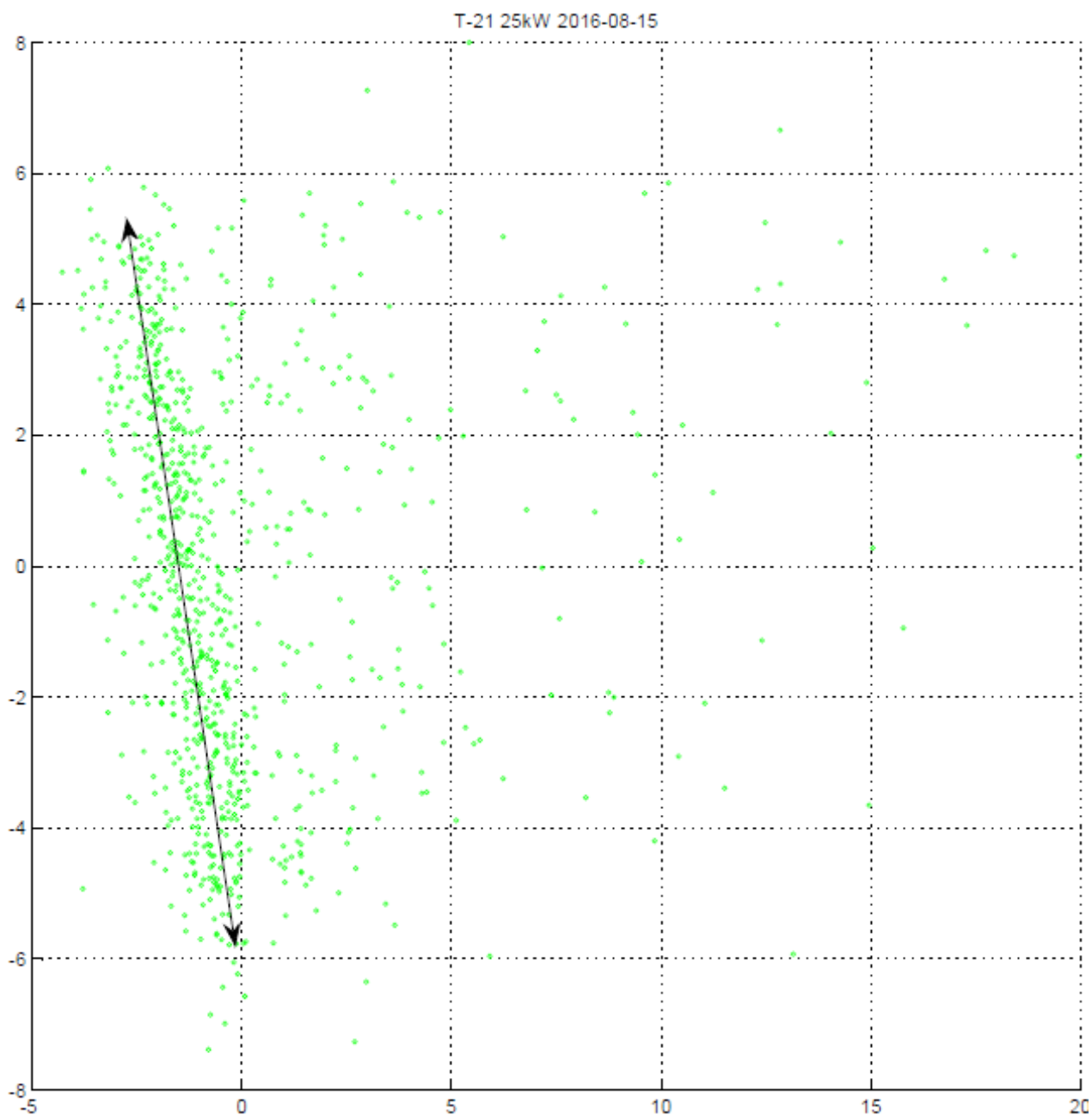
3.2.1 Pav. T-21 25 kW duomenų atvaizdavimas dvimatėje plokštumoje pasinaudojus Sammon algoritmu
