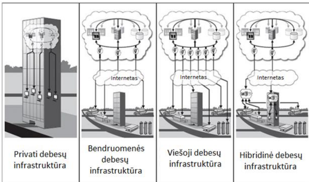
2.2.2 Pav. Debesų kompiuterijos išdėstymo modeliai
