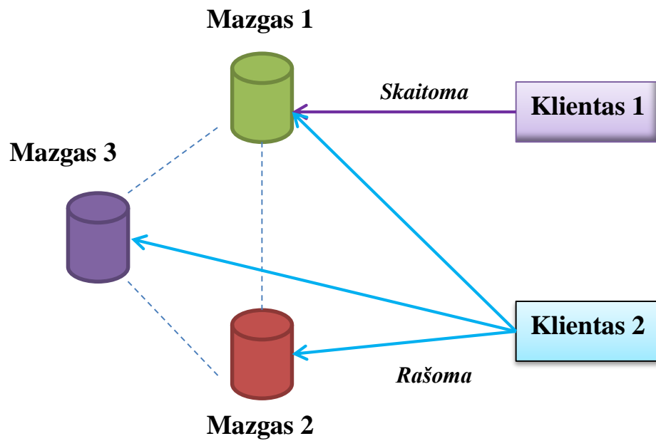
2.5.2 Pav. NoSQL duomenų bazės sistemos modelis skaitant ir rašant įrašus
