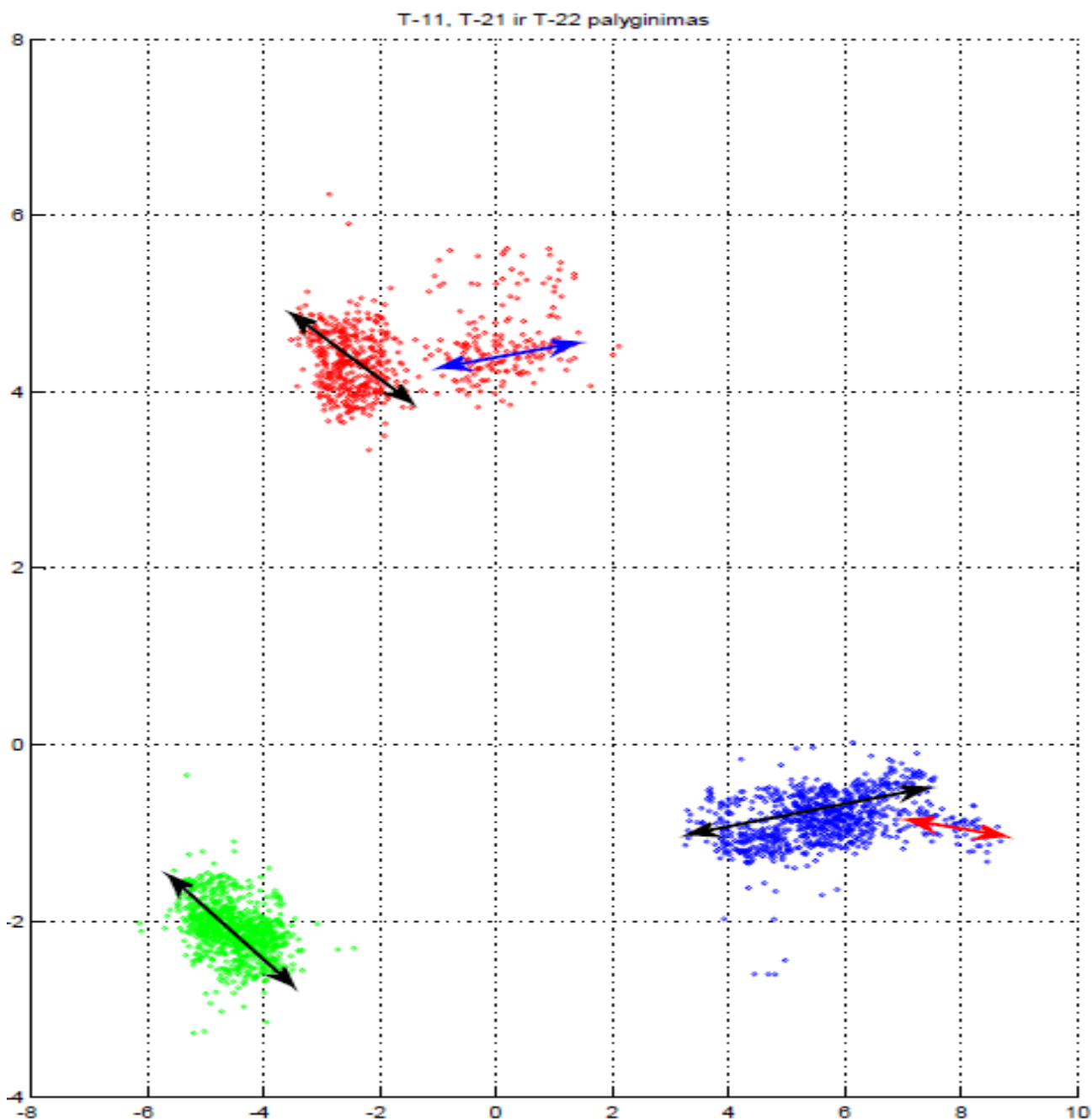
3.2.4 Pav. Savų reikmių transformatorių duomenų atvaizdavimas dvimatėje plokštumoje pasinaudojus Sammon algoritmu
