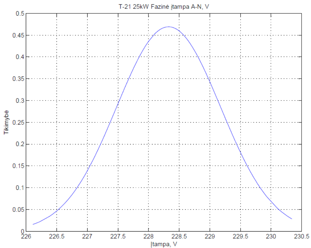
4.2.2 Pav. T-21 25 kW savų reikmių transformatoriaus normalusis (Gauso) skirstinys
