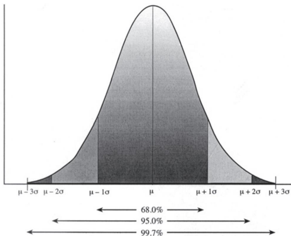
4.1.1 Pav. Normalusis (Gauso) skirstinys
