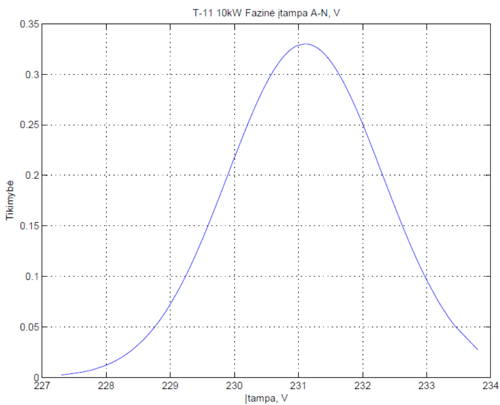
4.2.1 Pav. T-11 10 kW savų reikmių transformatoriaus normalusis (Gauso) skirstinys
