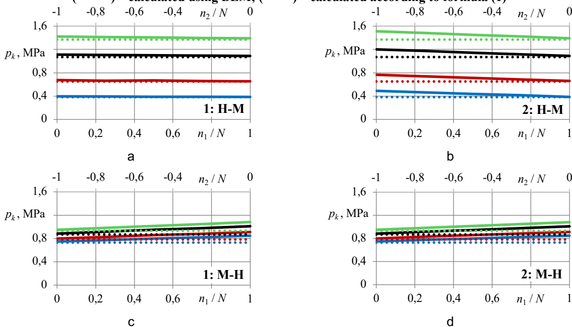
6 Fig. Kontaktnio slėgio p_k priklausomybė nuo nuokrypių n_1 ir n_2 bei išorinio sluoksnio storio s_2 , kai: p_0 = 0 ; N = 0.077 mm; d_2 = 14 mm; s_1 = 0.5 mm; ■ – s_2 = 0.3 mm; ■ – s_2 = 0.5 mm; ■ – s_2 = 0.8 mm; ■ – s_2 = 1.0 mm; a – 1-o modelio H-M tipas; b – 2-o modelio H-M tipas; c – 1-o modelio M-H tipas; d – 2-o modelio M-H tipas; (—) – apskaičiuota taikant BEM; (····) – apskaičiuota pagal (1) formulę
