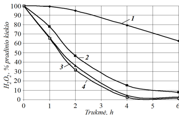
1 pav. Vandenilio peroksido skilimo vandeninėje terpėje priklausomybė nuo trukmės, kai naudojamo katalizatoriaus \text{Mn}^{2+} jonų koncentracija: 1 – be katalizatoriaus; 2 – 14 \mu\text{mol/L} ; 3 – 28 \mu\text{mol/L} ; 4 – 56 \mu\text{mol/L} . Terpės pH 9,0 \pm 0,2 ; temperatūra 20 \pm 1 °C
